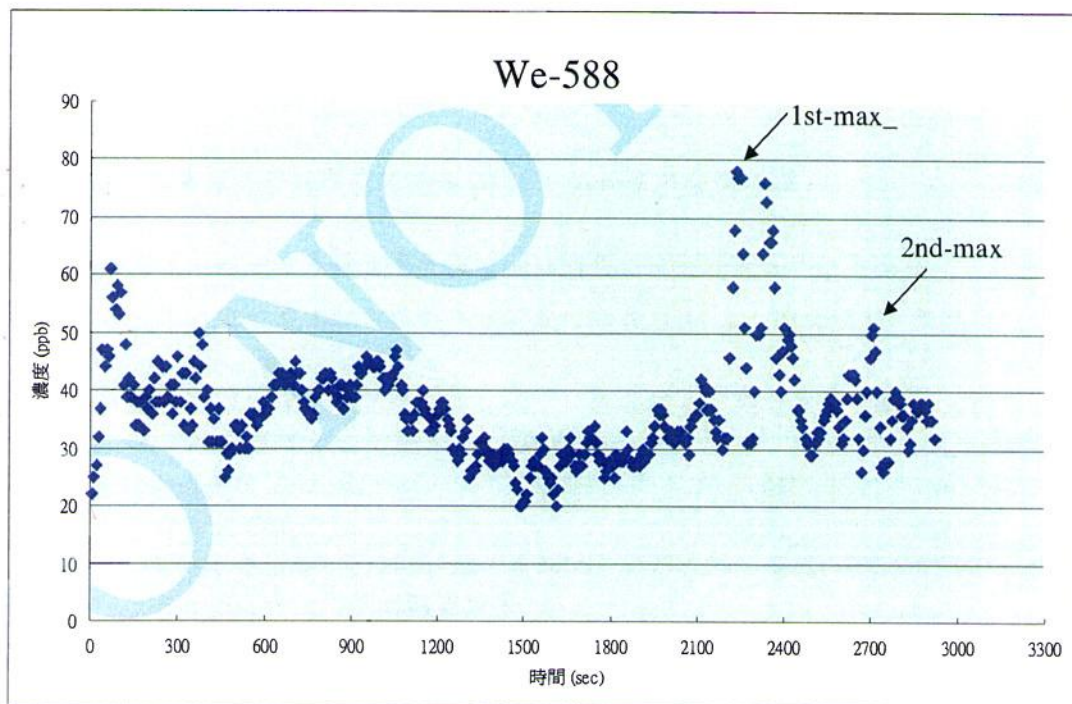
圖五 採樣時之臭氧濃度變化
